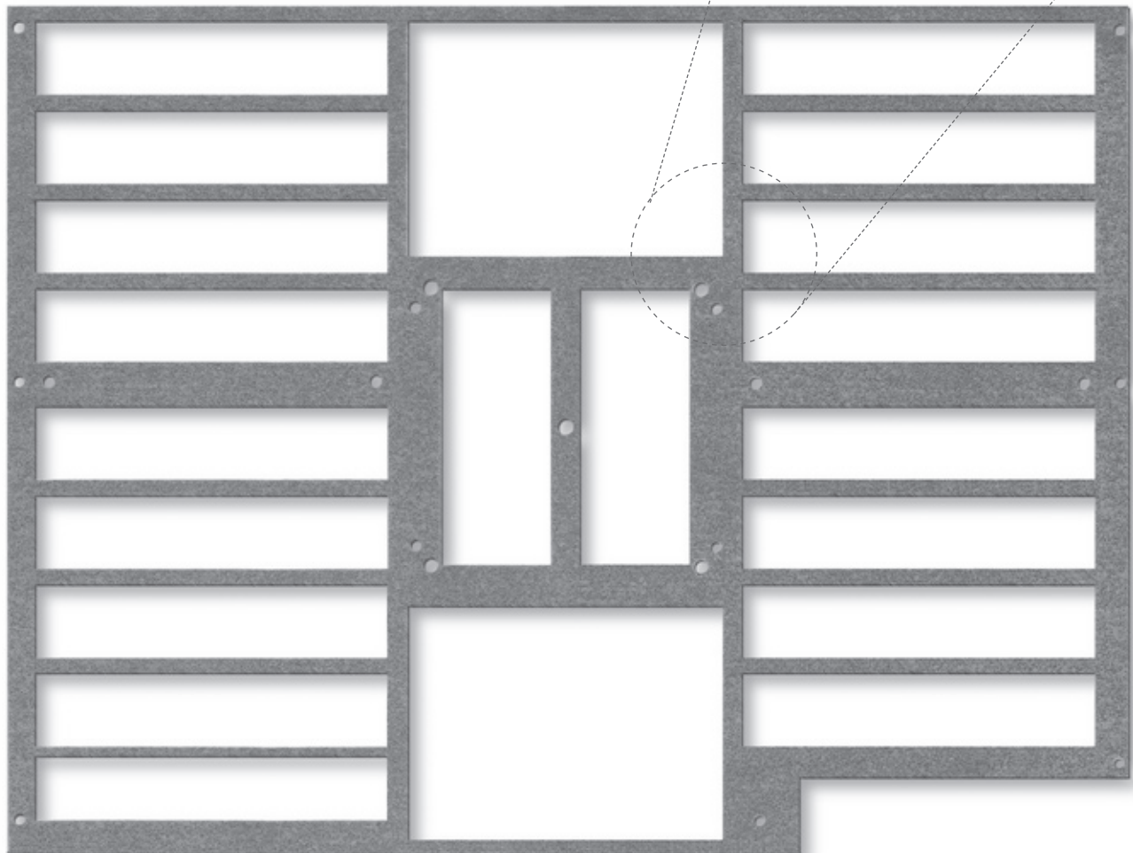
Precision die cut gasket - 15" x 12"
